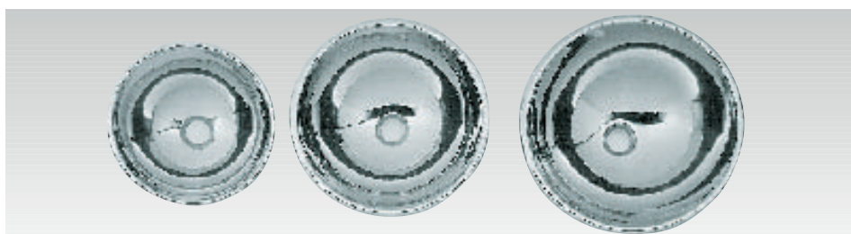
KO-28 Lavabo inox Ø interior 265 mm. Ø exterior 305 mm. KO-37 Lavabo inox Ø interior 315 mm. Ø exterior 355 mm. KO-39 Lavabo inox Ø interior 355 mm. Ø exterior 405 mm.
